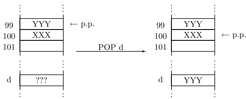
Figura 3.5. Interpretación gráfica de la orden POP.
