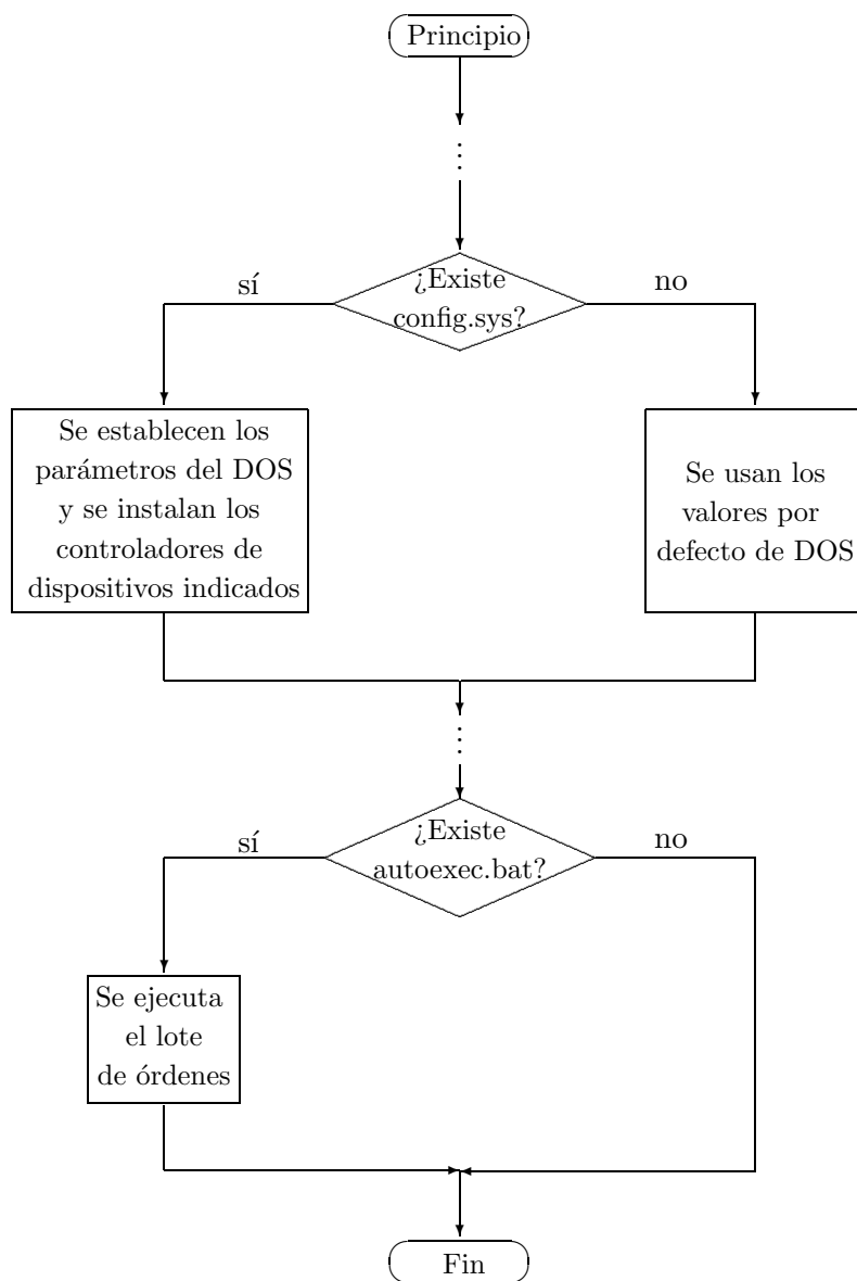
Figura A.3. Diagrama de flujo del arranque de DOS.
